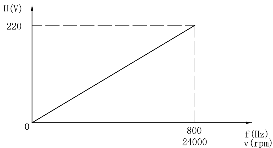
U. f Curve
