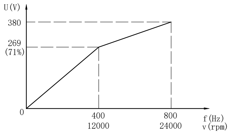
U. f Curve
