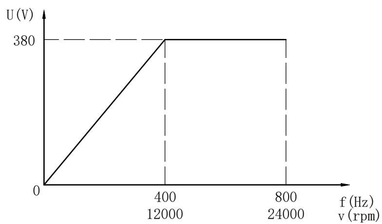
U. f Curve
