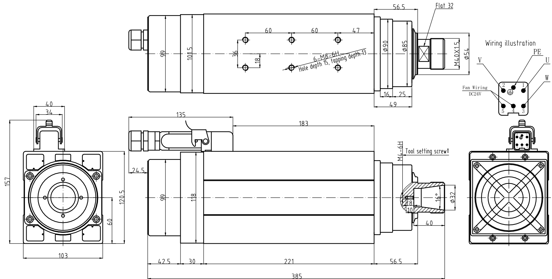
GDF60-18Z/5.5 380V外形图
