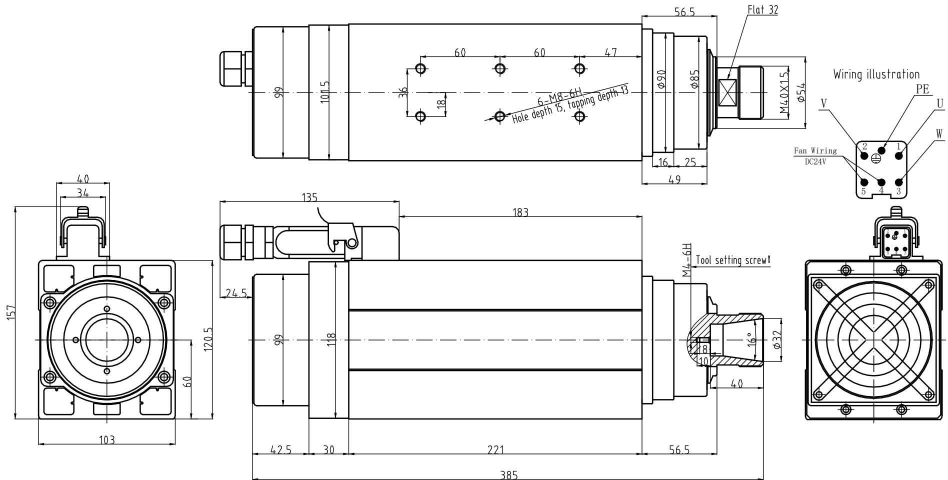
GDF60-18Z/5.5 220V外形图
